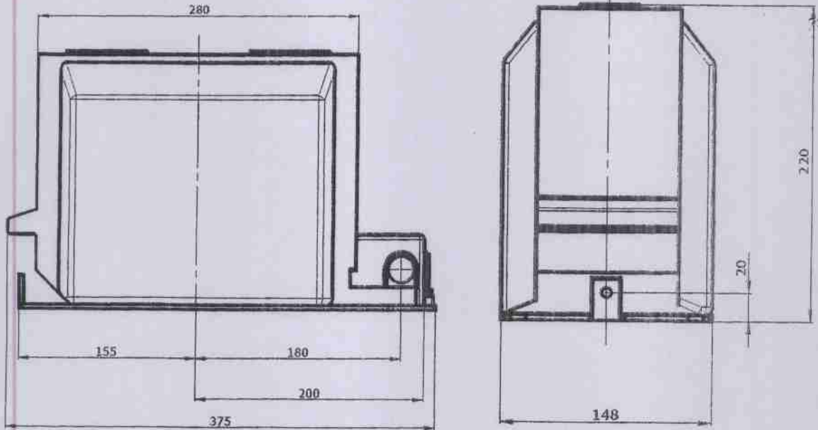
DFM – 24 feszültségváltó körvonalrajzai
